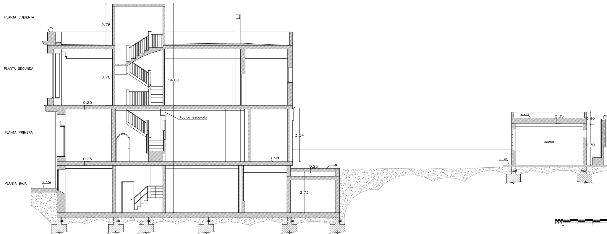
SECCION LONGITUDINAL
