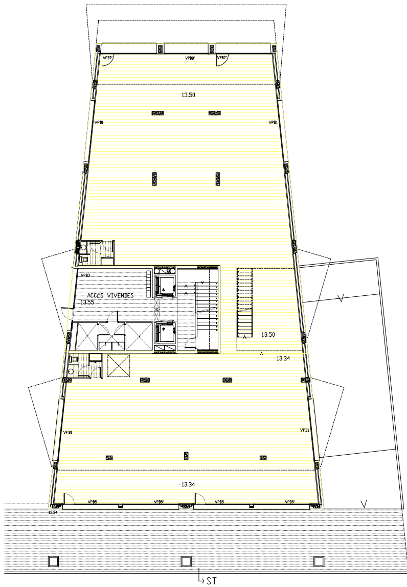
PLANTA BAJA
